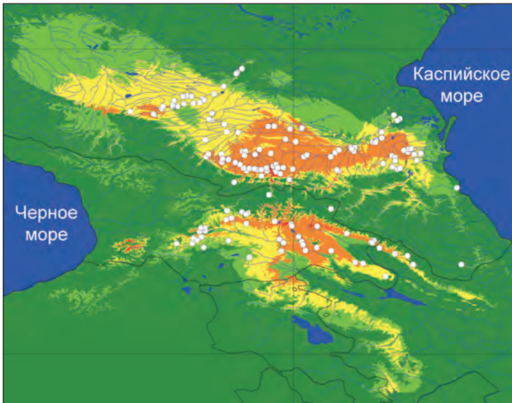
Рис. 1. Карта прогнозируемой области географического распространения Darevskia p. praticola на Кавказе, построенная с применением программы Maxent 3.3.3к: ● – высокая (100 – 74%), ● – средняя (74 – 56%), ● – низкая вероятность (56 – 37%) – предполагаемые подходящие территории; белые точки – места находок
