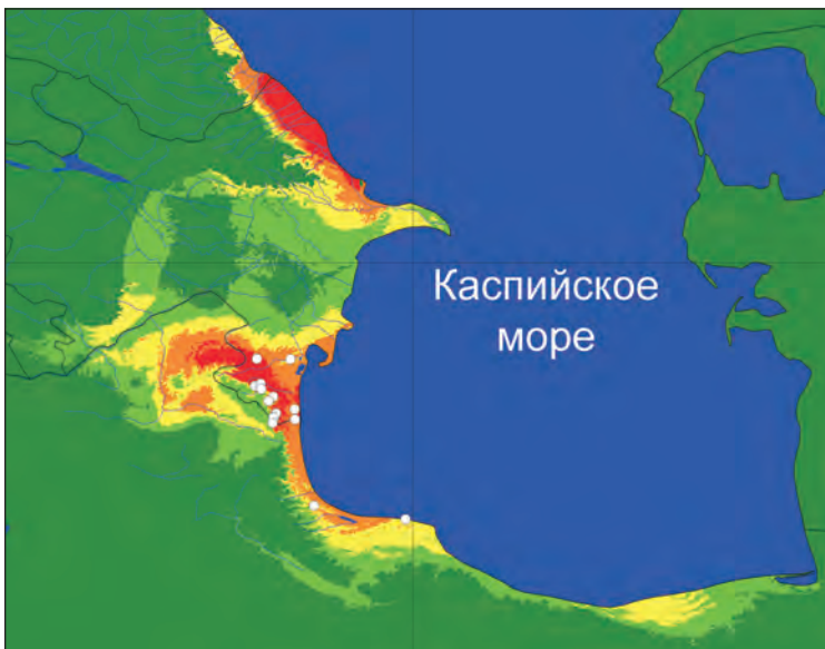
Рис. 2. Карта прогнозируемой области географического распространения Darevskia p. hyrcanica на Кавказе, построенная с применением программы Maxent 3.3.3к. Условные обозначения см. рис. 1
