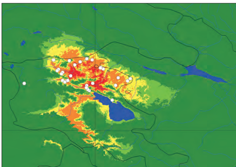
Рис. 4. Карта прогнозируемой области географического распространения Darevskia p. loriensis на Кавказе, построенная с применением программы Maxent 3.3.3k. Условные обозначения см. рис. 1
